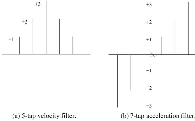
Fig. 13.7 FIR filters
