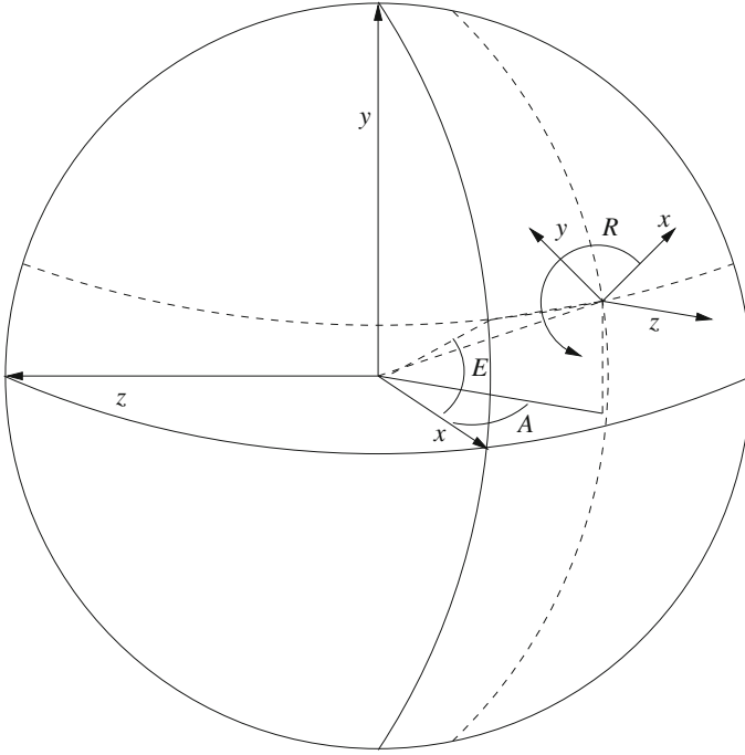
Fig. 7.3 Euler angles
