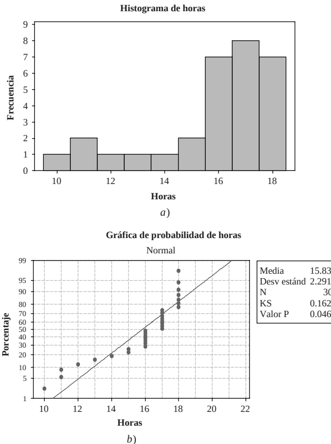
Figura 7-16 Prueba de Kolgomorov-Smirnov para normalidad; valor p = 0.046 , datos no normales.
