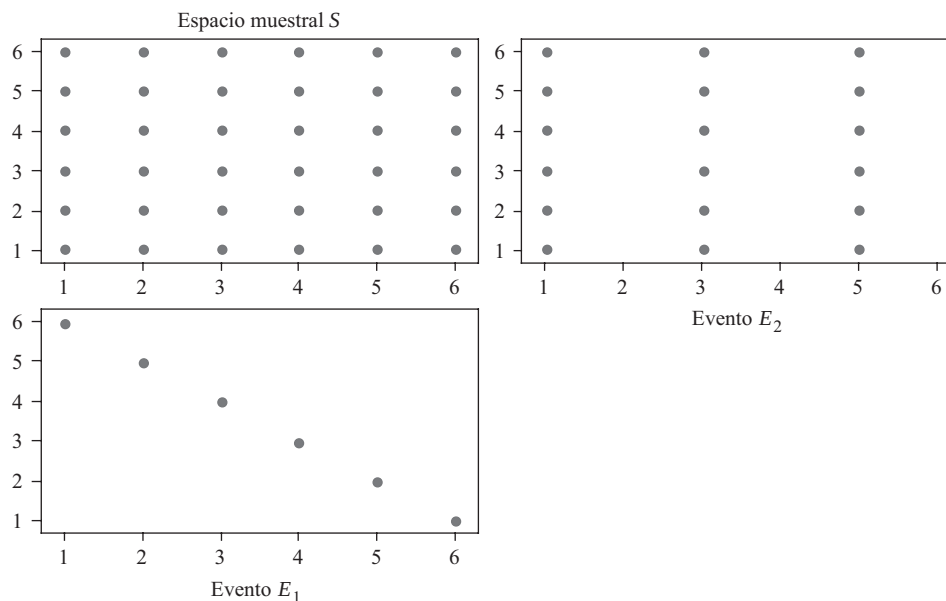
Figura 6-6 Resultados de MINITAB para el ejemplo 14.
