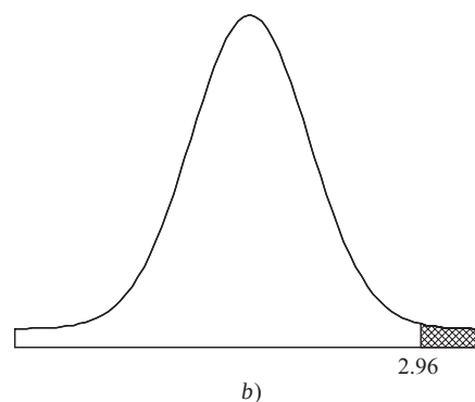
Figura 8-3 Las probabilidades muestrales se encuentran como áreas bajo la curva normal estándar.
