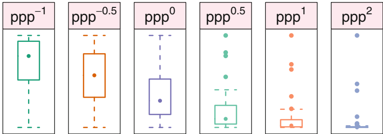
a. boxplots
